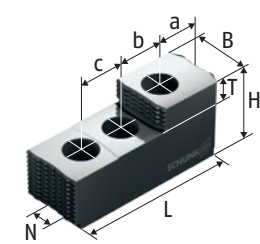
SP-HB-M/4 台阶式硬顶爪
