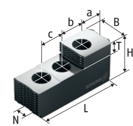
SP-HB-M/4 台阶式硬顶爪
