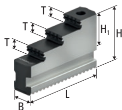
STF Mors durs étagés monoblocs
