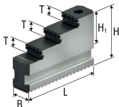
STF Tvrdé stupňovité monoblokové čelisti
