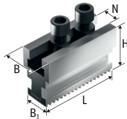
STB-G Ganasce base
