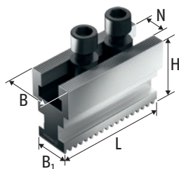
STB-G Základné čeľuste
