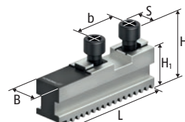
GBK Szczęki bazowe
