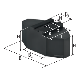
SWB-SM Segmentové čeľuste
