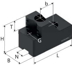
SZA 嵌入爪
