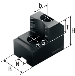
SZA 嵌入爪
