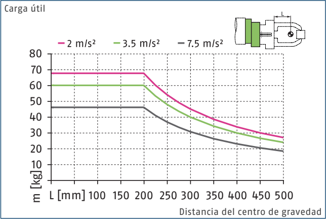
Diagrama de carga – diseño horizontal, no centrado (memoria de posición)
