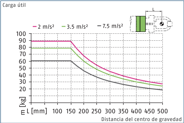
Diagrama de carga – diseño horizontal, centrado
