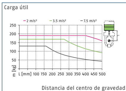
Diagrama de carga – diseño vertical, no centrado (memoria de posición)
