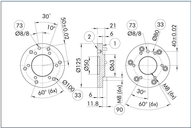
Адаптерная плита A-ISO080/ISO100
