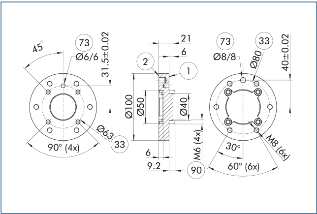
Адаптерная плита A-ISO080/ISO063
