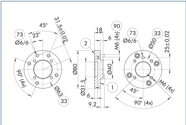
Адаптерная плита A-ISO050/ISO063
