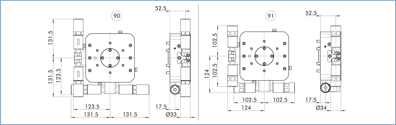
90 Пружинный патрон (FP) 91 Накачной патрон (LP)
