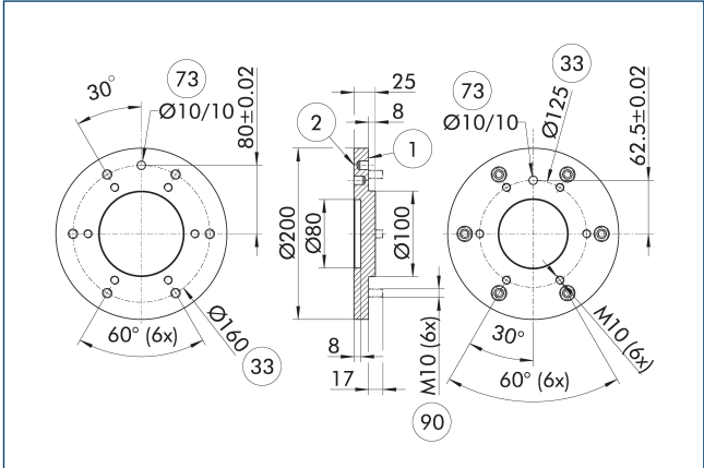
Адаптерная плита A-ISO125/ISO160
