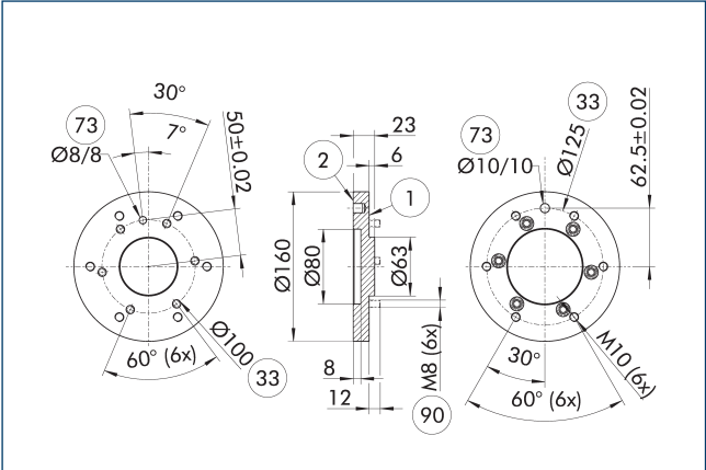
Адаптерная плита A-ISO125/ISO100
