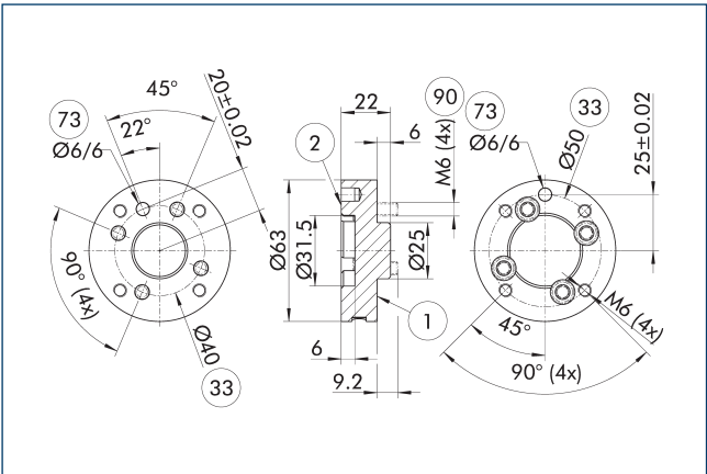
Адаптерная плита A-ISO050/ISO040
