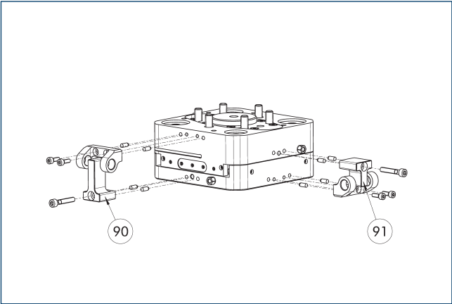
90 Комплект для присоединения, длинный 91 Комплект для присоединения, короткий
