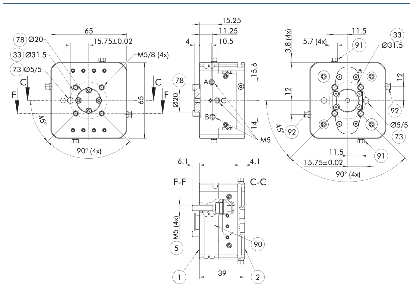
主视图 AGM-XY 031
