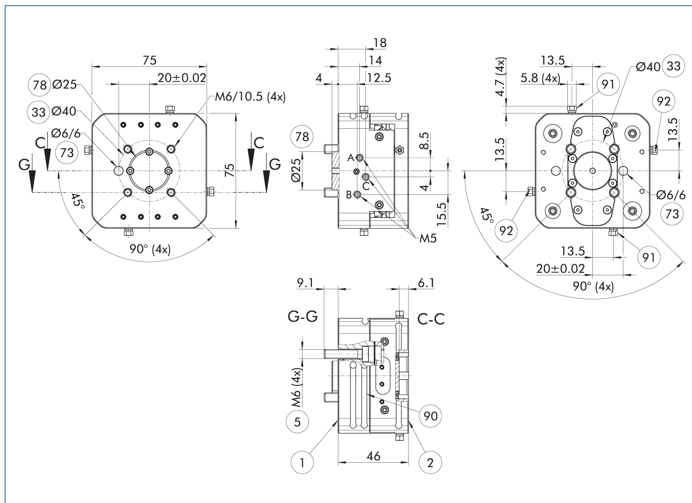
主视图 AGM-XY 040
