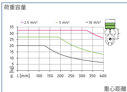
荷重線図 - 垂直セットアップ、非中心配置 (ポジションメモリ)
