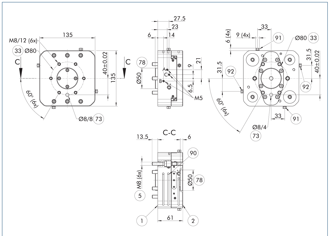
主视图 AGM-XY 080
