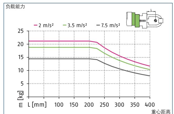
负载图 — 水平结构，偏心（位置存储器）
