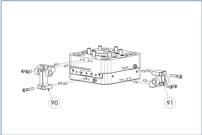
90 Set di montaggio, lungo 91 Set di montaggio, corto
