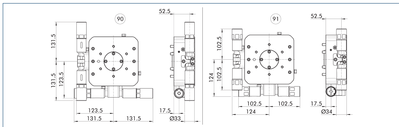
90 Cartuccia a molla (FP)
