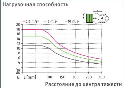
Диаграмма нагрузки: горизонтально, заблокировано
