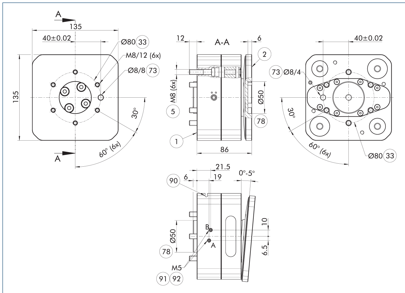
主视图 AGM-W 080
