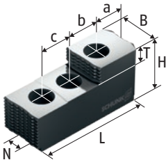
SP-HB 台阶式硬顶爪
