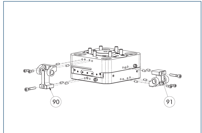
90 Anbausatz lang
