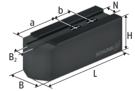
KM-WBL Morsetti riportati teneri
