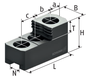
SHB-J Harde, vertande bovenste klemmen
