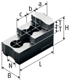
SHB Harde, vertande bovenste klemmen
