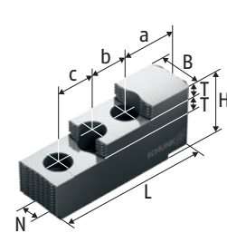
SP-HB 台阶式硬顶爪
