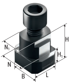
NS T 型螺母
