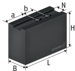
SWB 软顶爪
