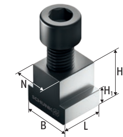
NKS T 型螺母
