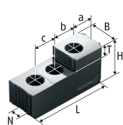
SP-HB Закаленные ступенчатые накладные кулачки
