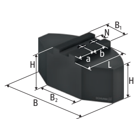
SWB-SM Сегментные кулачки
