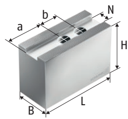
SWB-AL ソフトトップジョー
