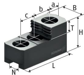
SHB-J 台阶式硬顶爪
