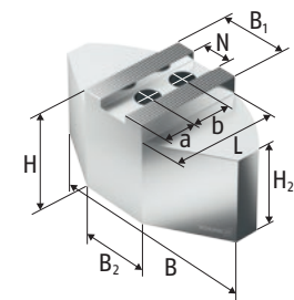
KMWB-SA 阶梯夹爪
