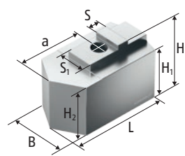
SRK-AL 软顶爪
