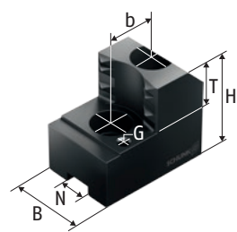
SZ4 嵌入爪
