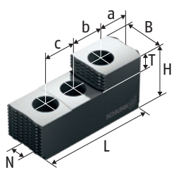
SP-HB 台阶式硬顶爪
