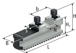
SFGF-K Základné čeľuste
