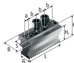
STNJ Базовые кулачки
