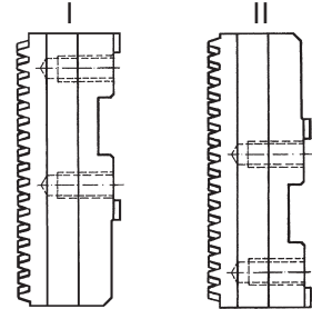
基爪位置
