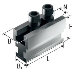
STB-G 基爪
