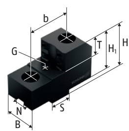
SZKA 嵌入爪
