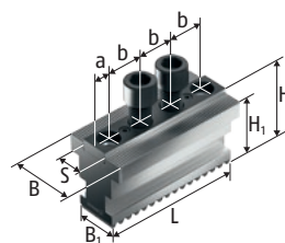
STNJ 基爪
