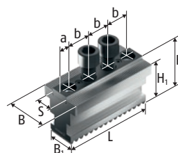
STN Базовые кулачки
