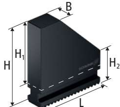
UVB-HS Mäkké monoblokové čeľuste
