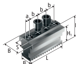
STNJ Základné čeľuste
