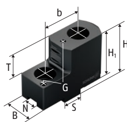
SZKU Univerzálne drapákové čeľuste
