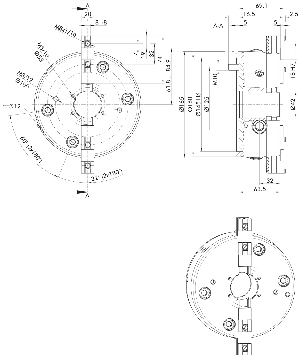
Mandrin de serrage de l'arbre tiré en position ouverte. Sous réserve de modifications techniques.
