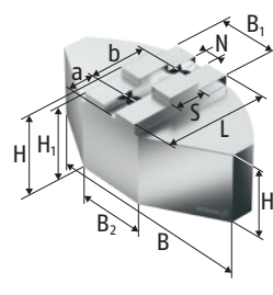
SFA-SA Morsetti avvolgenti
