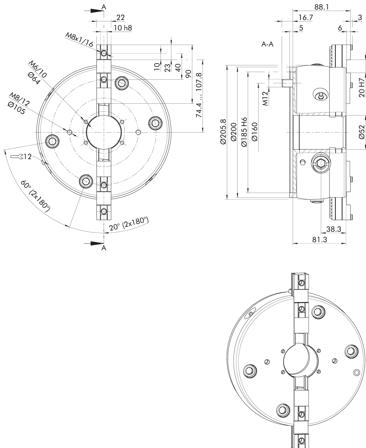
Mandrino per il bloccaggio dell'albero rappresentato in posizione aperta. Soggetto a modifiche tecniche.
