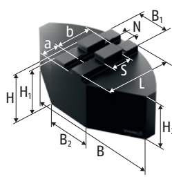
SFA-SM Morsetti avvolgenti
