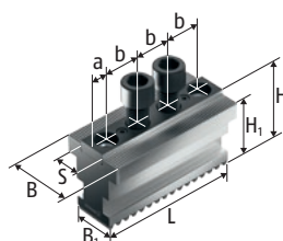
STN Ganasce base
