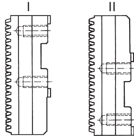
Positie van basisklemmen
