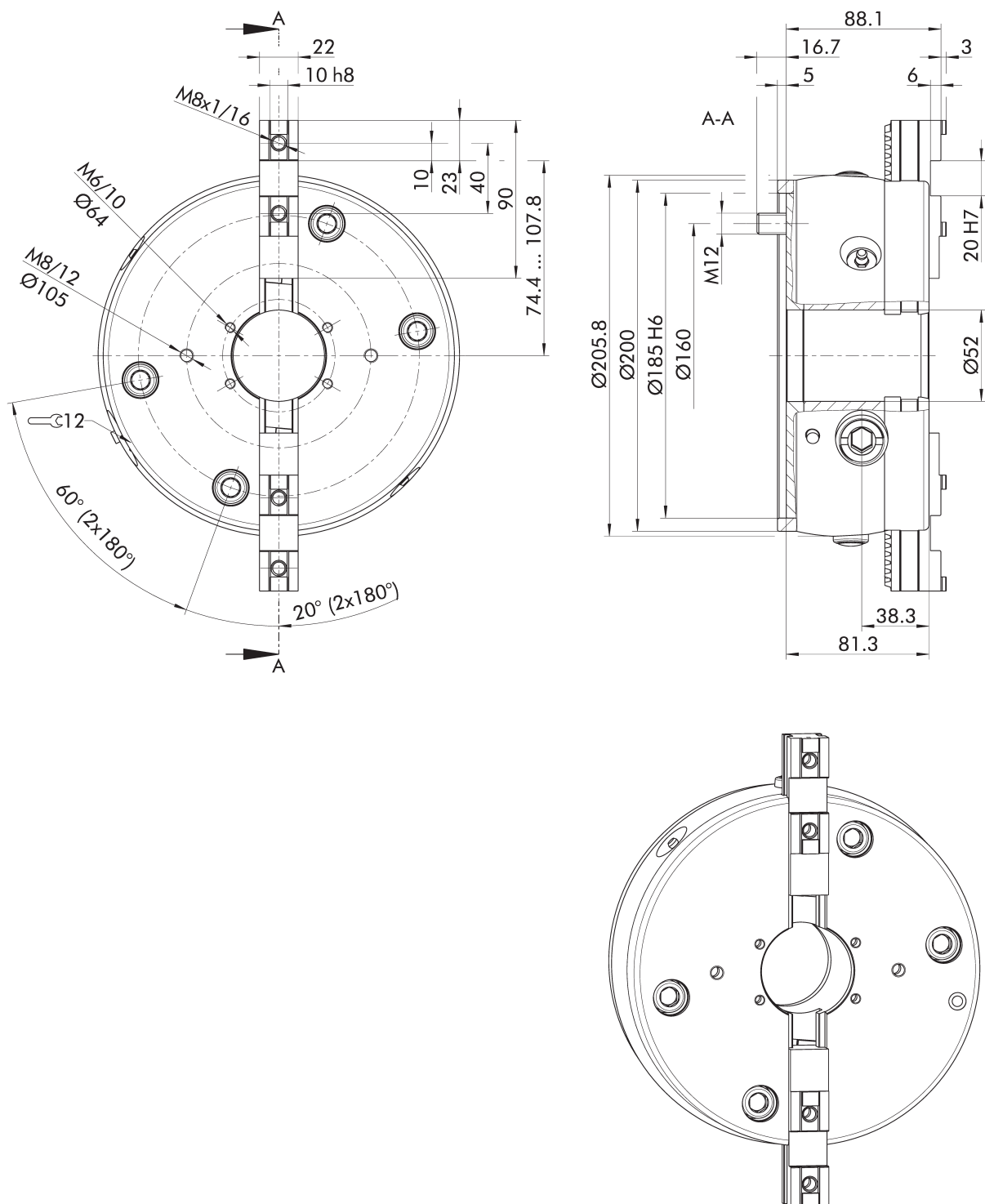
Klauwplaat voor klemming van de as, weergegeven in open positie. Technische wijzigingen voorbehouden.
