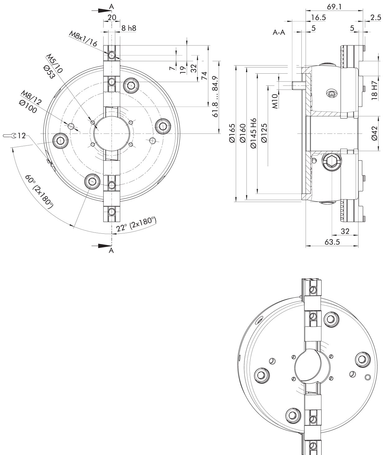
Klauwplaat voor klemming van de as, weergegeven in open positie. Technische wijzigingen voorbehouden.
