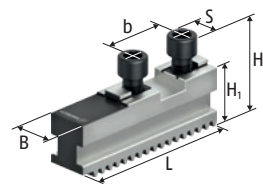
SFG 基爪
