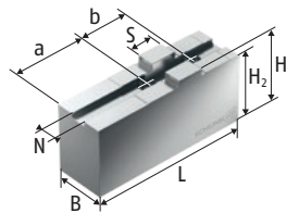
SFA-AL 软顶爪
