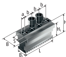
STN 基爪
