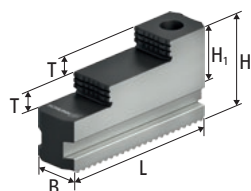
STF 台阶式硬整体爪
