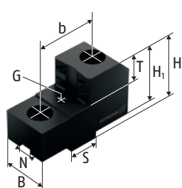
SZKA 嵌入爪
