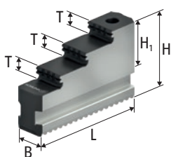
STF 台阶式硬整体爪
