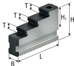
STF Закаленные ступенчатые блочные кулачки
