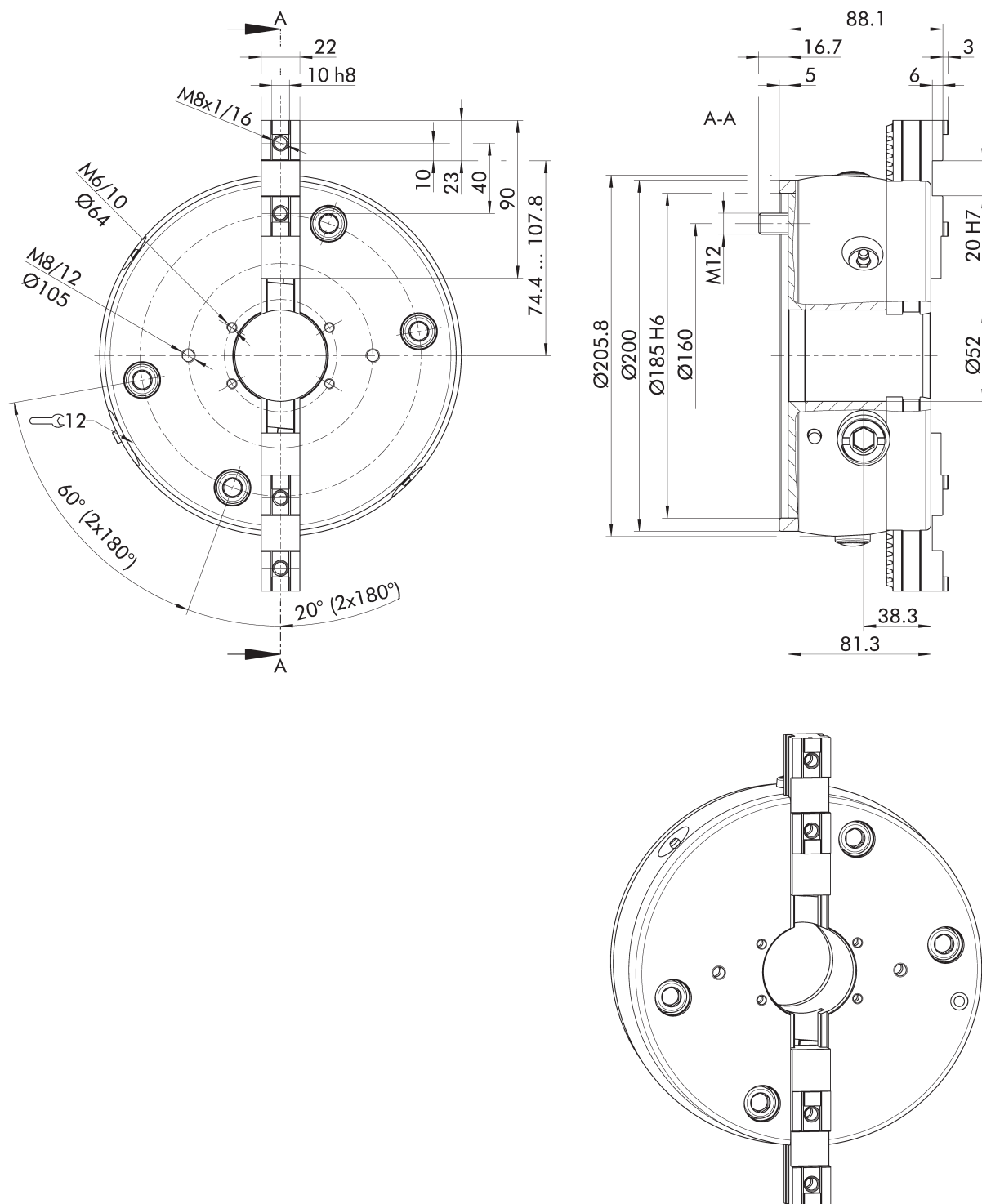
Mandrill para fixação do eixo puxado na posição aberta. Sujeito a alterações técnicas.
