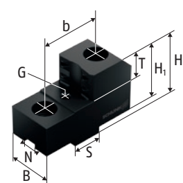
SZKA Зубчатые кулачки
