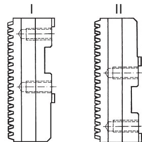
Положение базовых кулачков
