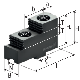
SHF Morsetti riportati a gradino rigidi
