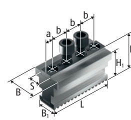
STNJ Ganasce base
