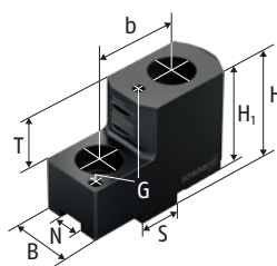
SZKU Universele klauwklemmen
