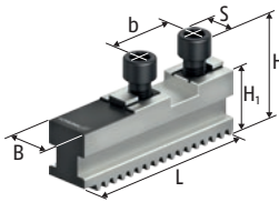
GBK Basisklemmen
