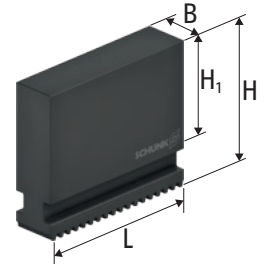
UVB Zachte monoblokklemmen
