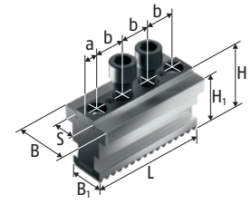
STNJ Basisklemmen
