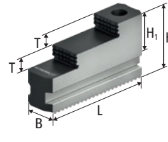
GST Harde, vertande blokklemmen
