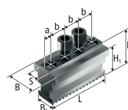
STNJ Szczęki bazowe
