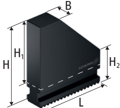
UVB-HS Szczęki jednolite, miękkie
