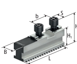
GBK Szczęki bazowe
