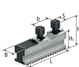
GST Tvrdé stupňovité monoblokové čelisti
