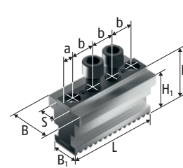
STNJ Základní čelisti
