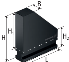
UVB-HS Měkké monoblokové čelisti
