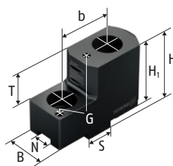
SZKU Univerzální hrubovací čelisti
