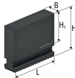
UVB ソフトモノブロックジョー
