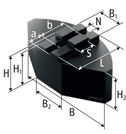
SFA-SM フルグリップジョー
