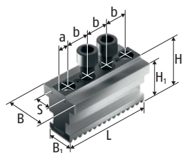
STN ベースジョー
