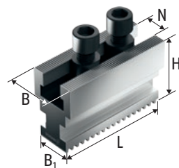
STB-G ベースジョー
